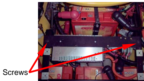
Remove DC-DC Converter If equipped
